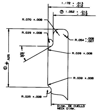
DETALLE DE CORONA FINISH DETAIL ESCALA 5:1 SCALE 5:1
